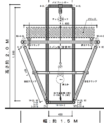
図1 簡易載荷試験装置
